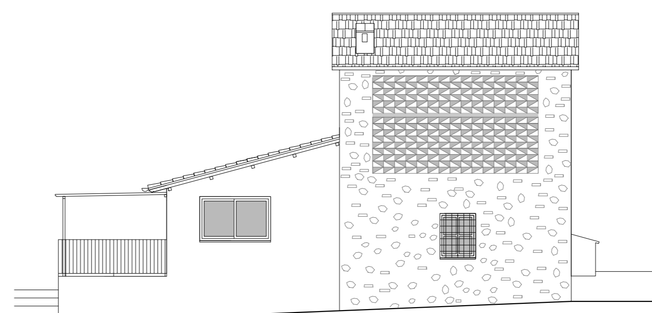
PROSPETTO SUD
