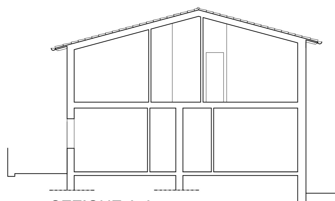
SEZIONE A-A
