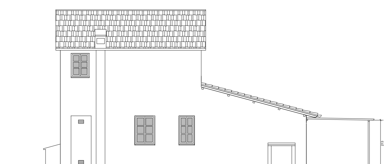
PROSPETTO NORD
