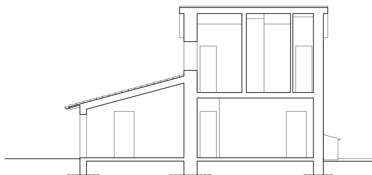
SEZIONE B-B
